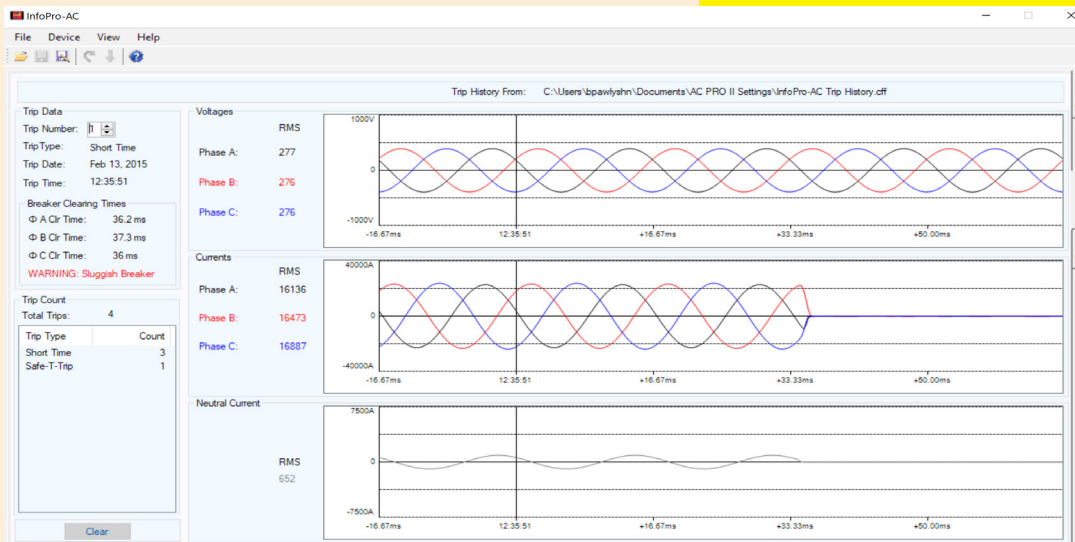
Pantalla de InfoPro con el historial de formas de onda de los disparos
